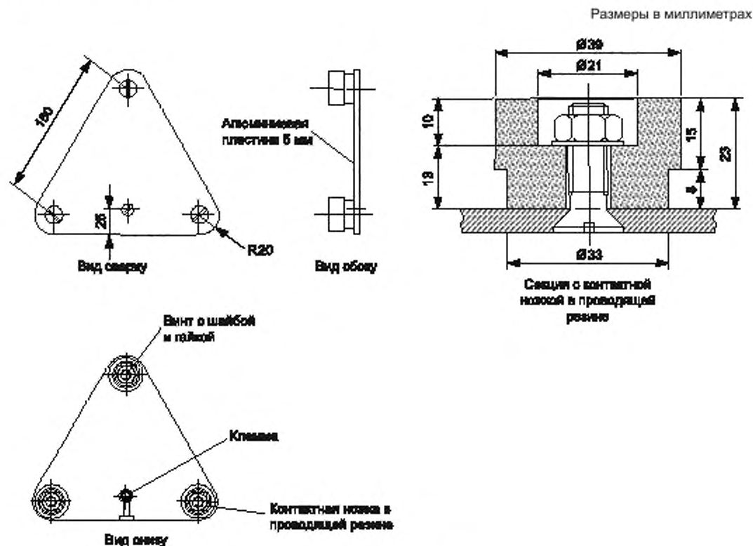
Рисунок В.1 — Испытательный электрод 1
