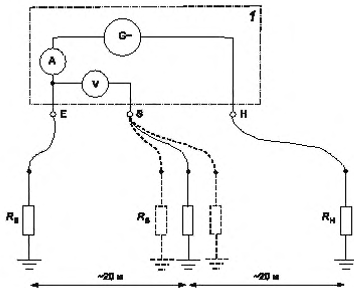
а) Линейное расположение электродов
