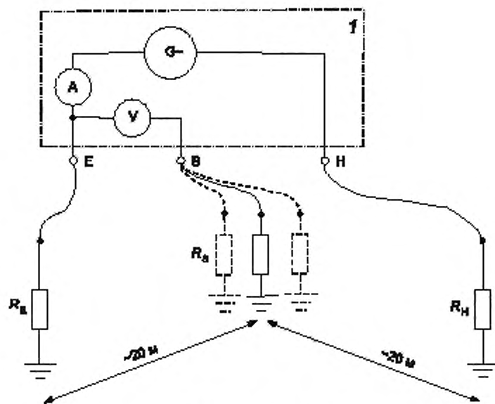
б) Расположение электродов треугольником
