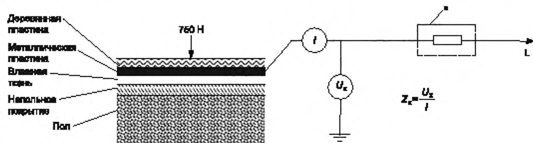
Рисунок В.2 — Испытательный электрод 2
